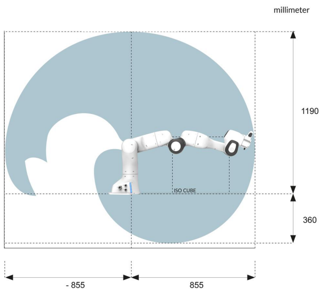
侧视图：末端执行器法兰的可达空间
